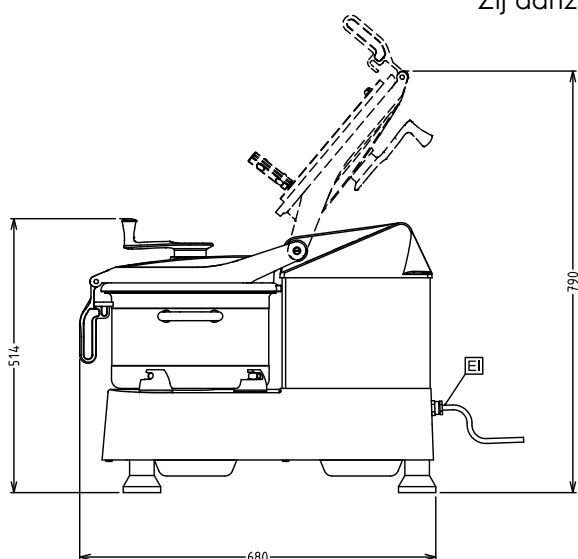
Zij aanzicht
